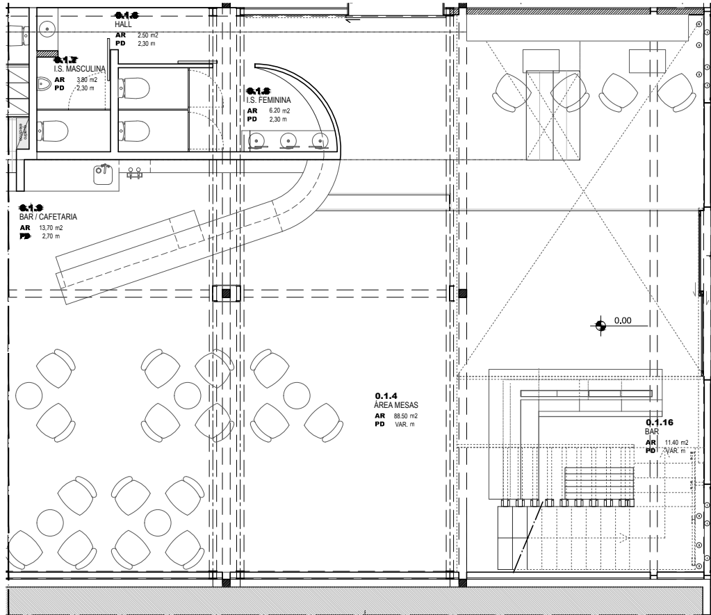
PLANTA PISO 0 | ESC. 1/100
