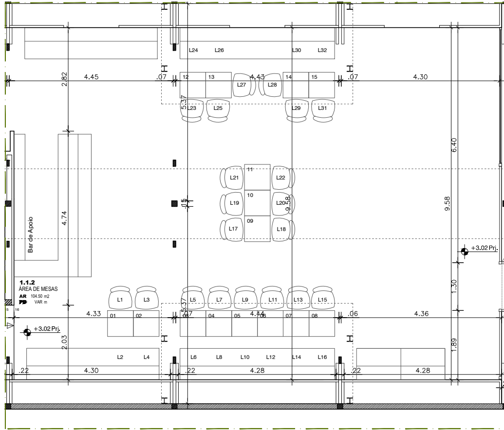
PLANTA PISO 1 | ESC. 1/100
